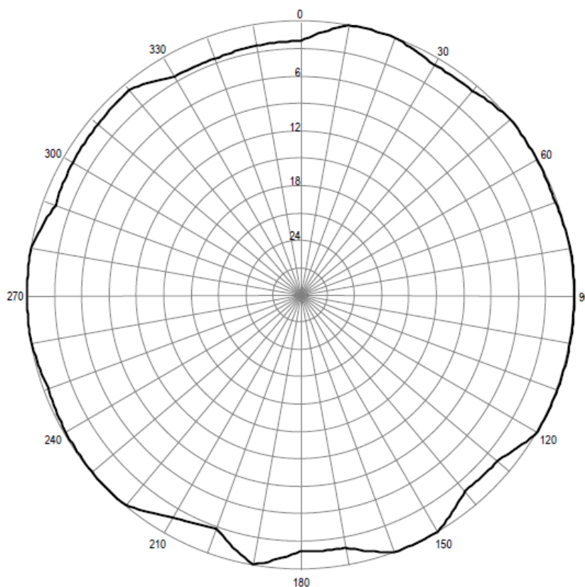
Pozioma charakterystyka promieniowania anteny stacji Warszawa Varso 89,80 MHz
